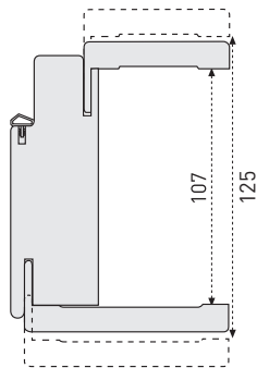
Telaio con coprifilo aletta lunga fino a 140 mm Frame with long-wing architrave up to 140mm
