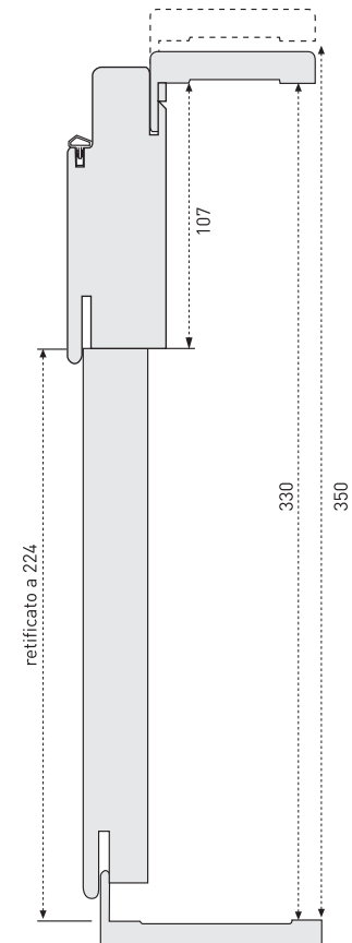
Telaio con foglio bussola fino a 350 mm Frame with socket sheet up to 350mm
